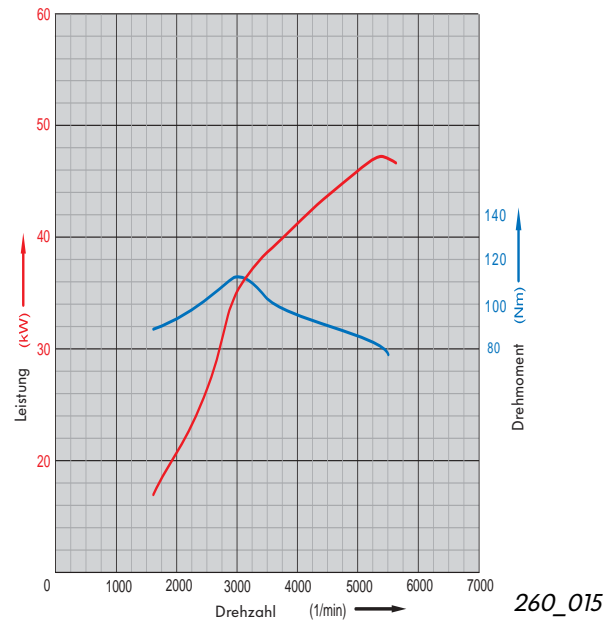
Leistungs- und Drehmomentkurve des 1,2l-12V-Motors
