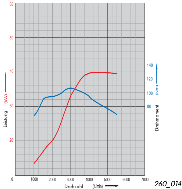
Leistungs- und Drehmomentkurve des 1,2l-6V-Motors
